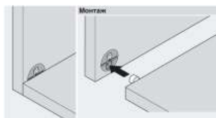
Стяжка с винтом
